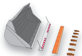
ERDSCHAUFEL
