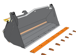
SCHAUFEL 4X1
